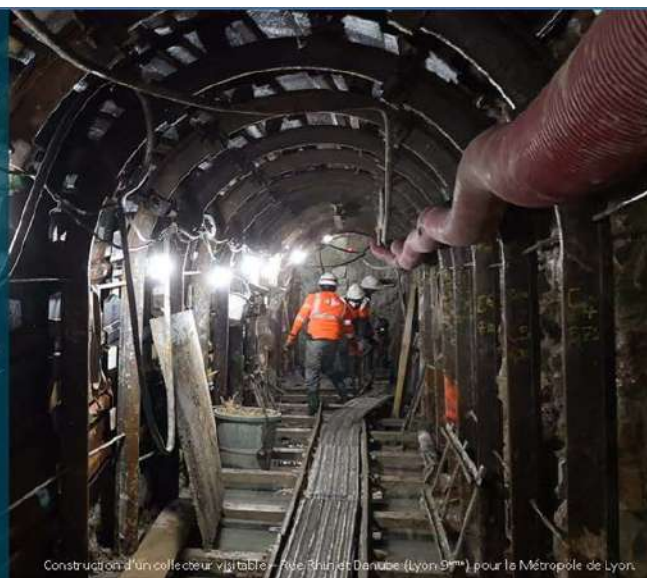
Construction d'un collecteur visitable - Rue Rhin et Danube (Lyon 9 ème ) pour la Métropole de Lyon.
